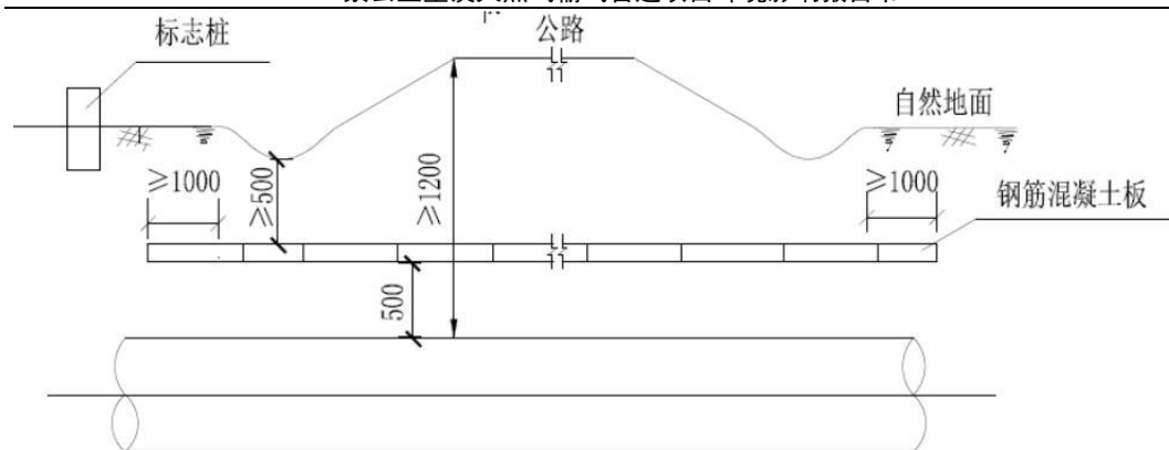
图3.1-8 开挖加盖板穿越断面典型示意图
