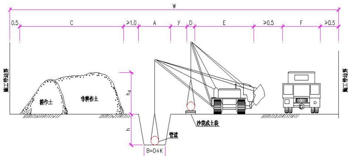
图3.1-2 施工作业带示意图
