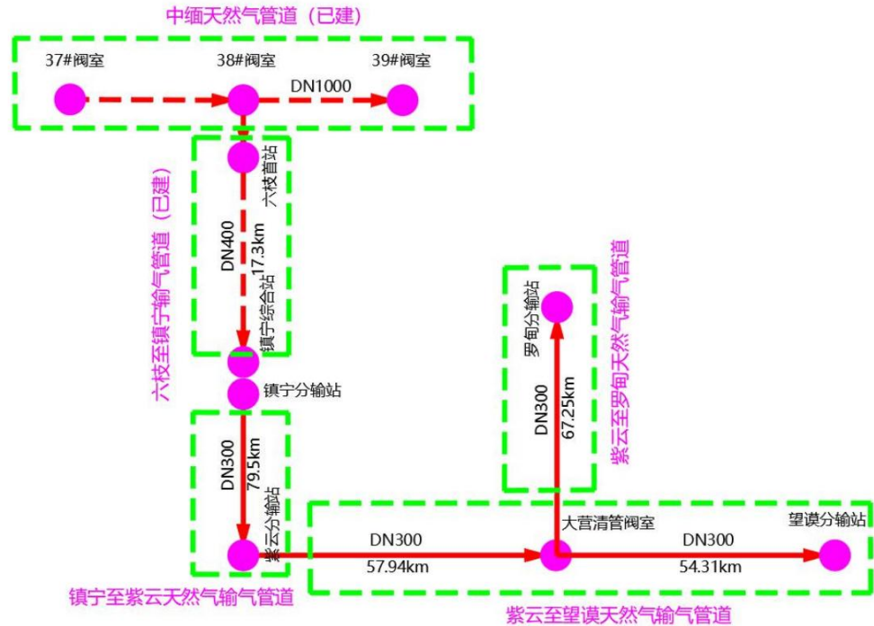
图2.2-2 全线工艺系统天然气流向图
