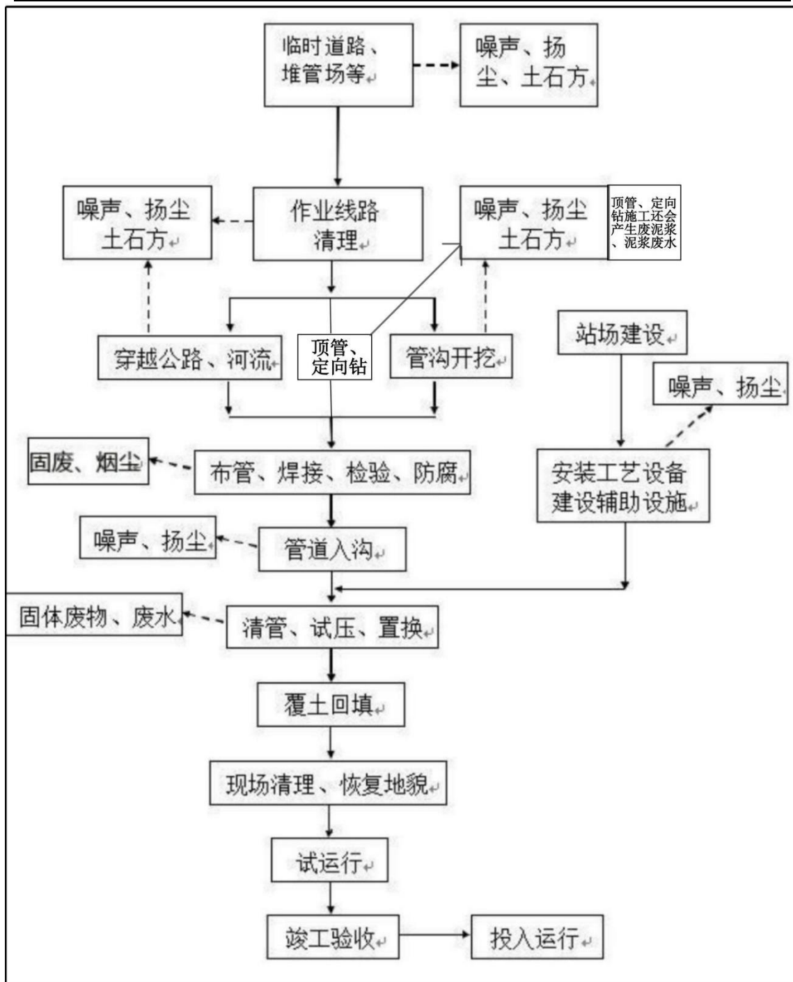
图3.1-1 项目施工工序及主要产污环节示意图
