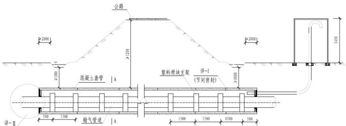
图3.1-7 套管穿越公路纵断面示意图
