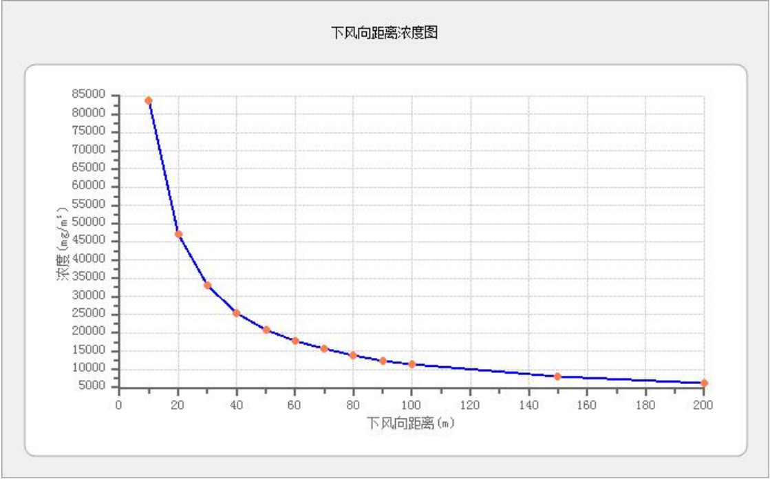
图 6.5-1 各管段泄露甲烷下风向不同距离处预测结果
