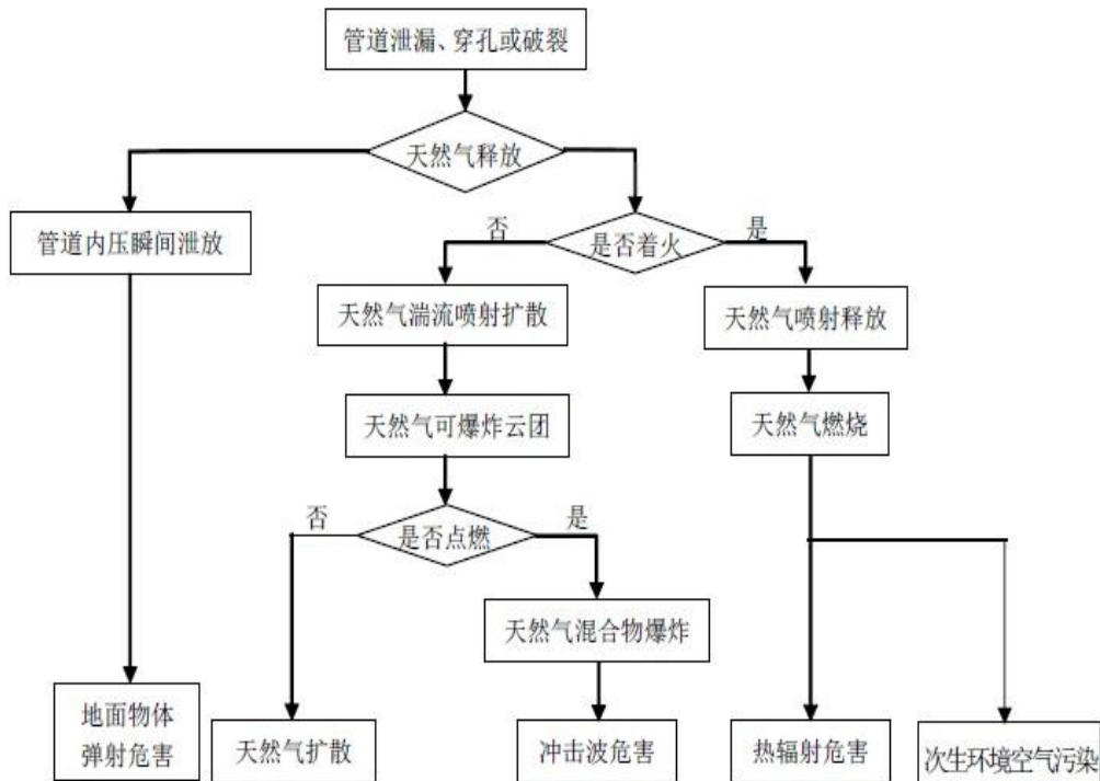
图 6.4-1 天然气管道事故树分析示意图
