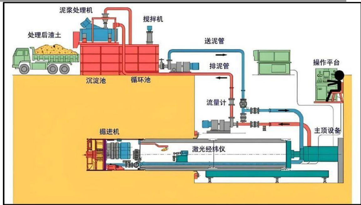
图3.1-6 顶管施工工艺示意图
