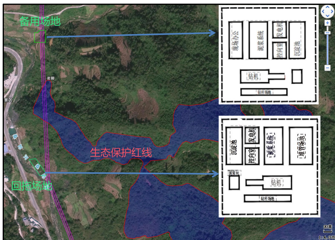
图2.4-9 定向钻穿越生态红线示意图
