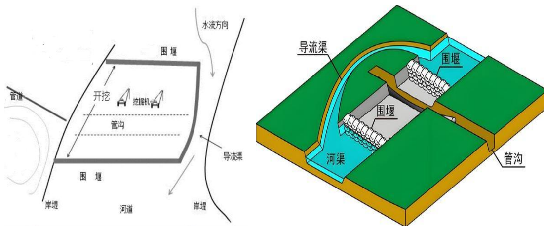
图3.1-5 围堰开挖作业带示意图
