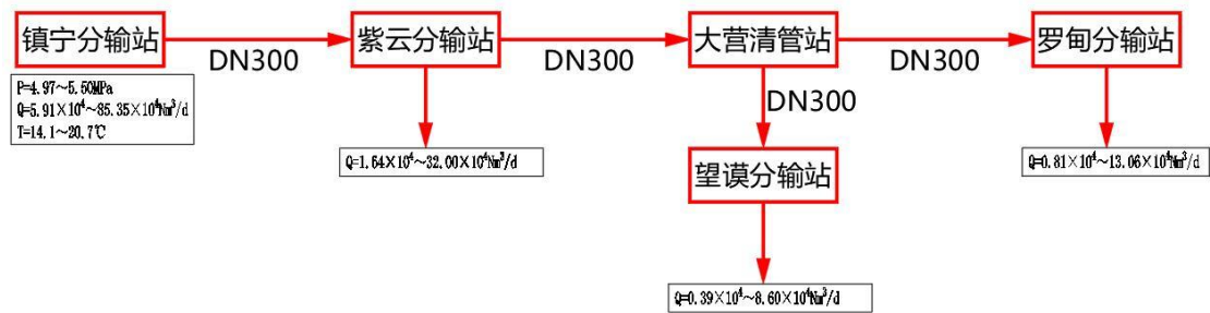
图2.2-2 输气工艺方案节点示意图
