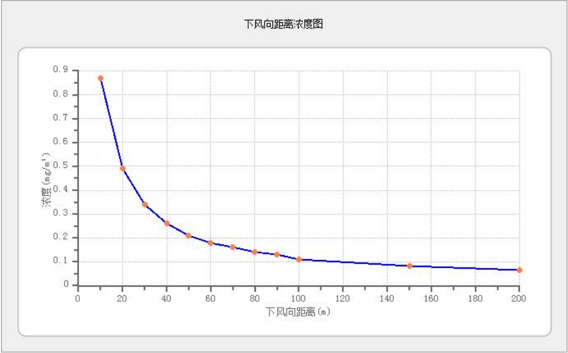
图 6.5-3 水塘阀室-猴场阀室段次生污染物 CO 下风向不同距离处预测结果
