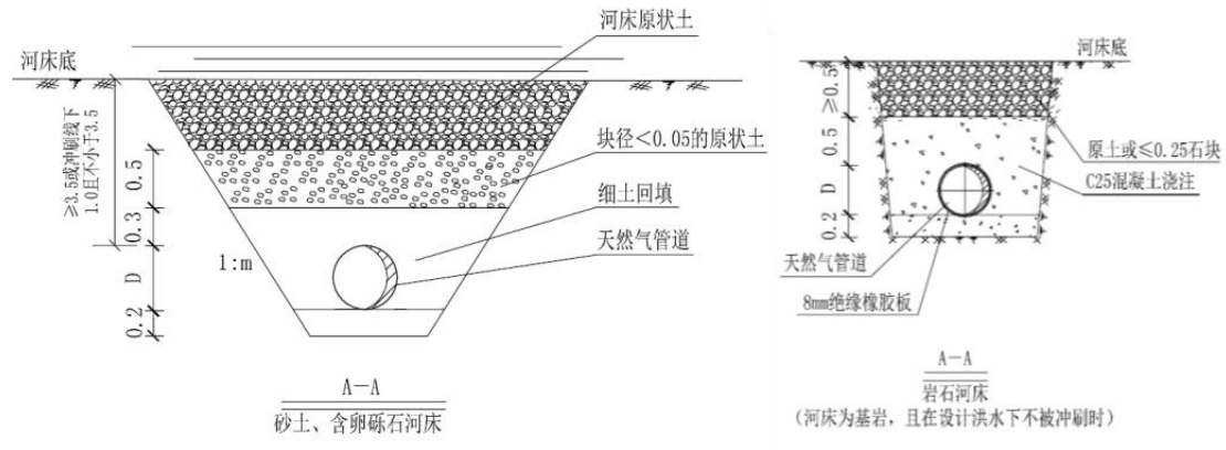
图2.4-8 大开挖穿越设计典型图
