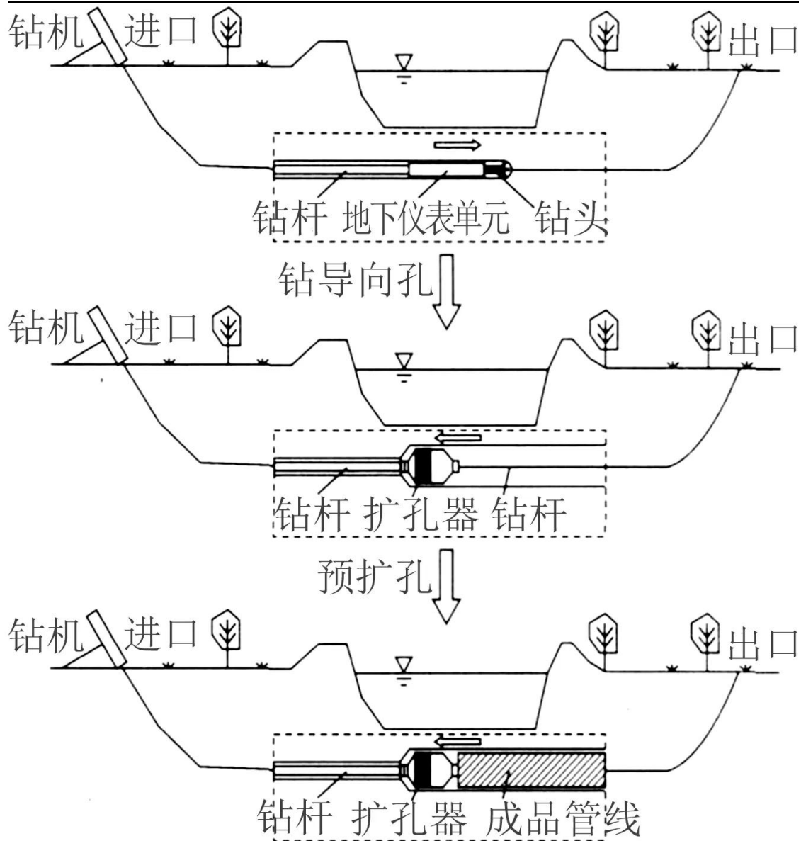
图3.1-3 定向钻穿越施工管线回拖过程断面示意图
