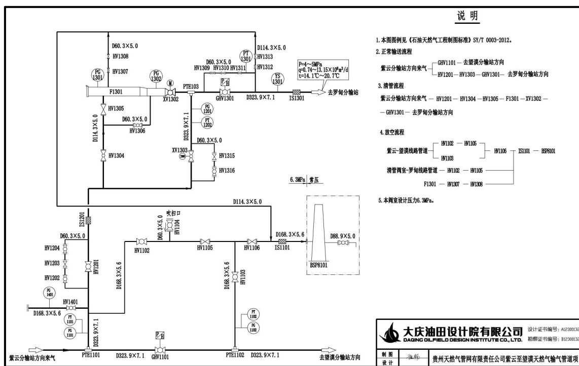
图 3.2-3 大营清管阀室工艺流程及产污节点图
