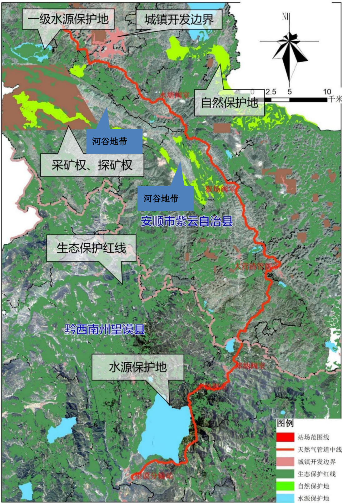
图 3.4-1 本工程管道整体走向示意图
